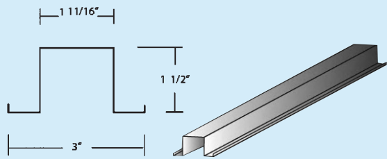
Hat Section
