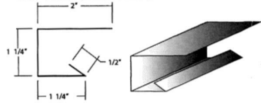
Jamb Trim (PBR-Panel)
