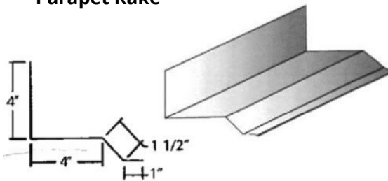
Parapet Rake
