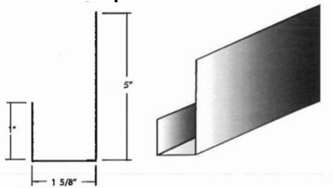
Fascia Wrap
